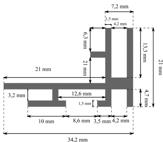
Przekrój techniczny profil CPA 21
